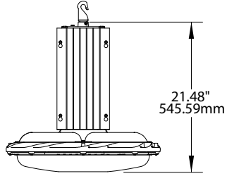
Pendant (PM)
